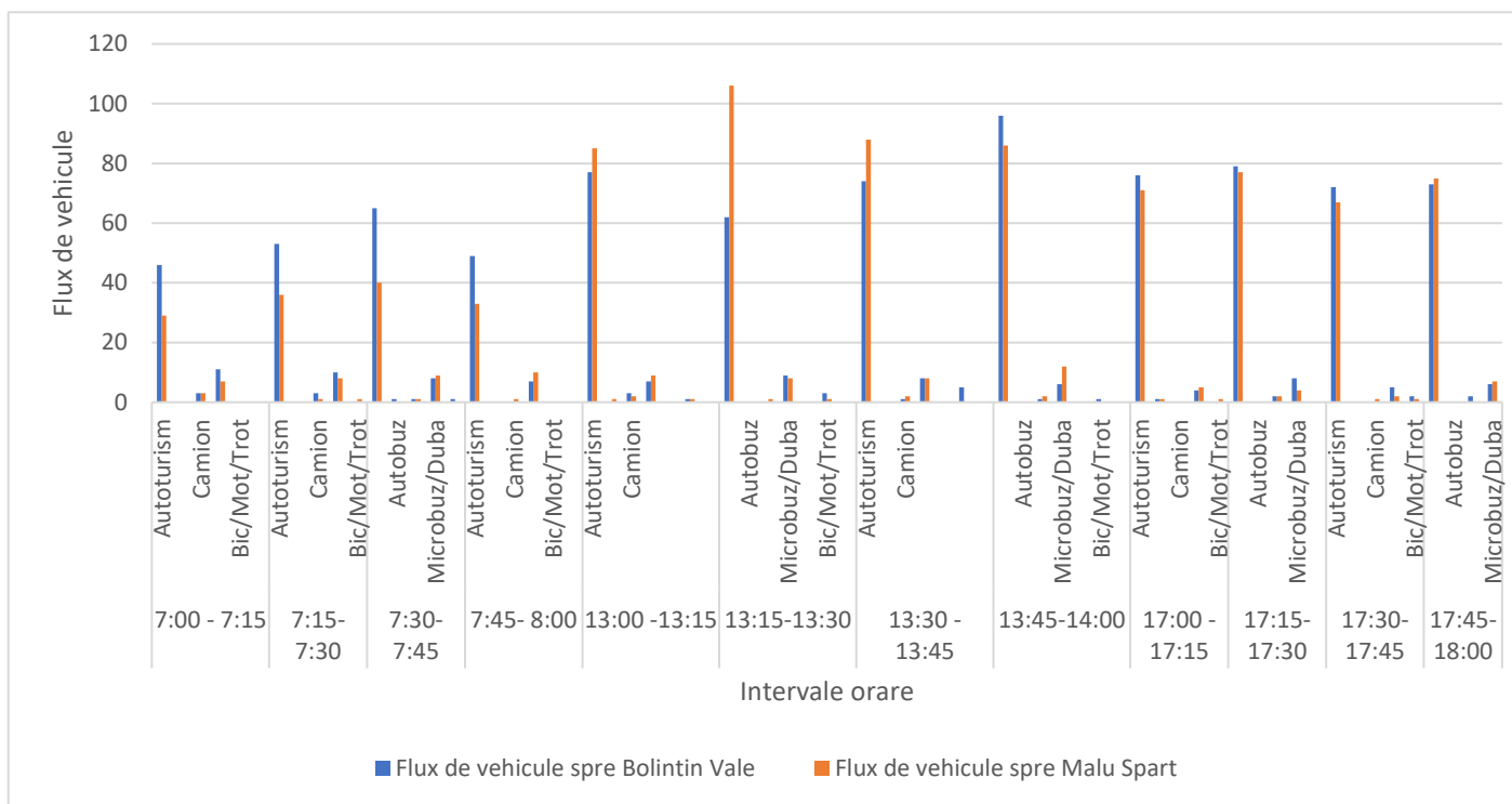
Fig. 3.2.19. Fluxul de vehicule care intră în Bolintin Vale și ies spre Malu Spart – DJ 610 (Camera 2.1.10)
