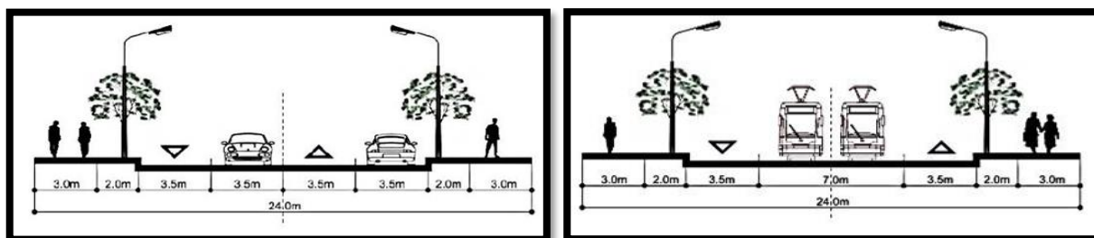
Fig.2.2.5 Profile, cu sau fără linii de tramvai, pentru străzile de categoria II – de legătură (sursa: [12])
