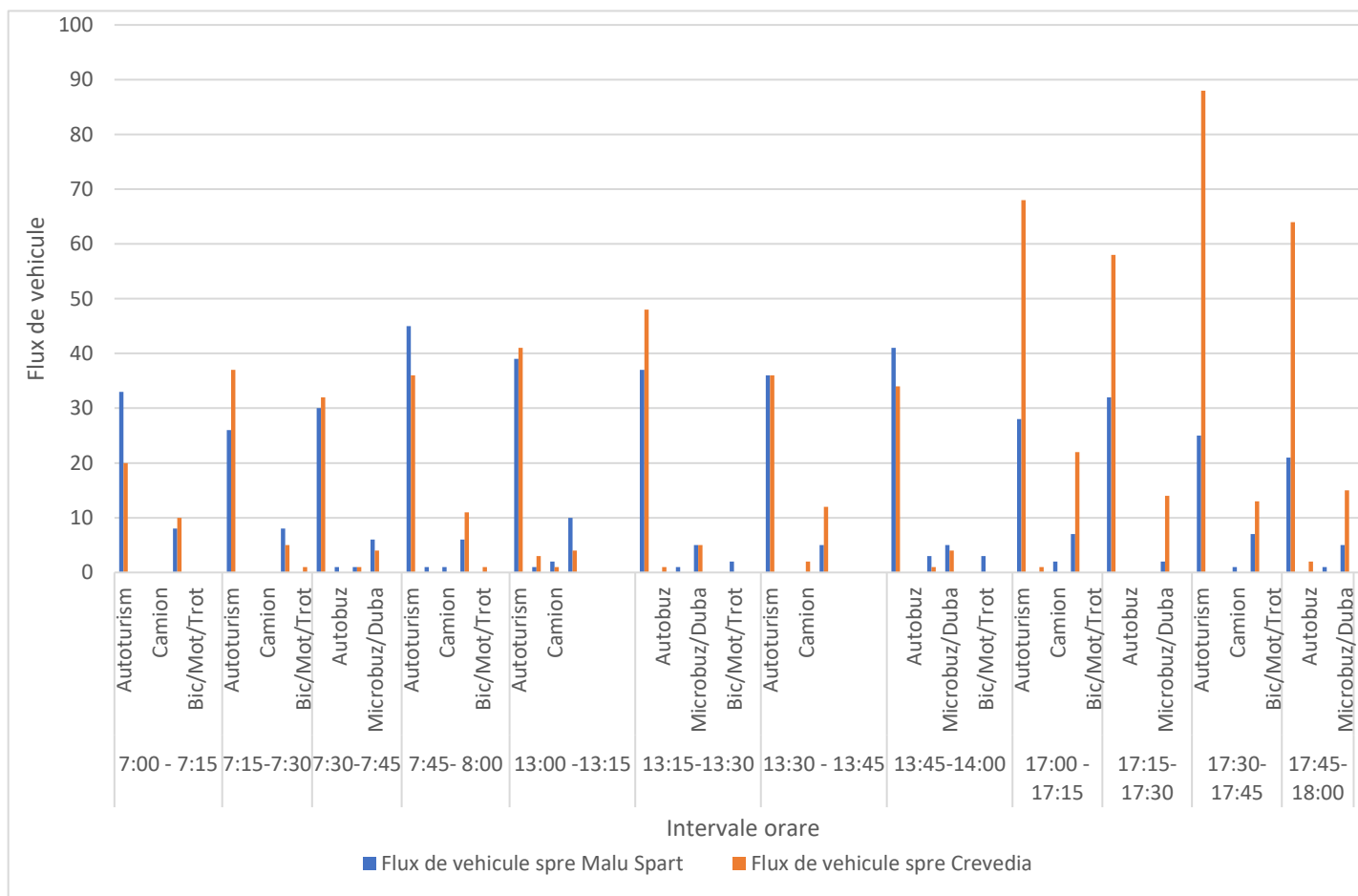
Fig. 3.2.22. Fluxul de vehicule ce se deplasează spre Malu Spart, respectiv Crevedia – punct de monitorizare Ocolul Silvic (Camera 2.3.2)
