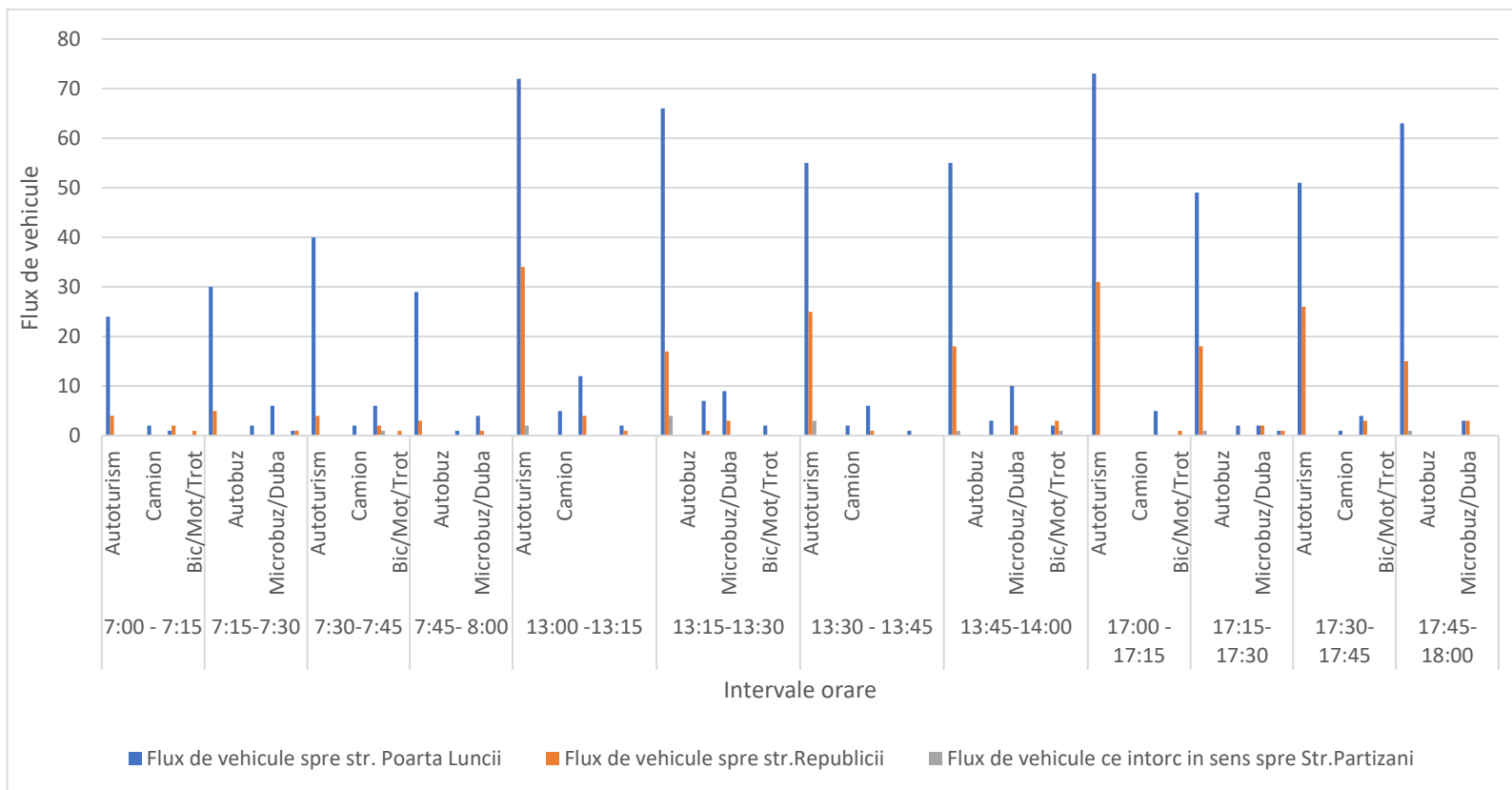
Fig. 3.2.17.c. Fluxul de vehicule care intră / ies în /din sensul giratoriu la intersecția străzilor Poarta Luncii, Partizani și Republicii – acces din strada Partizani (Camera 1.161)
