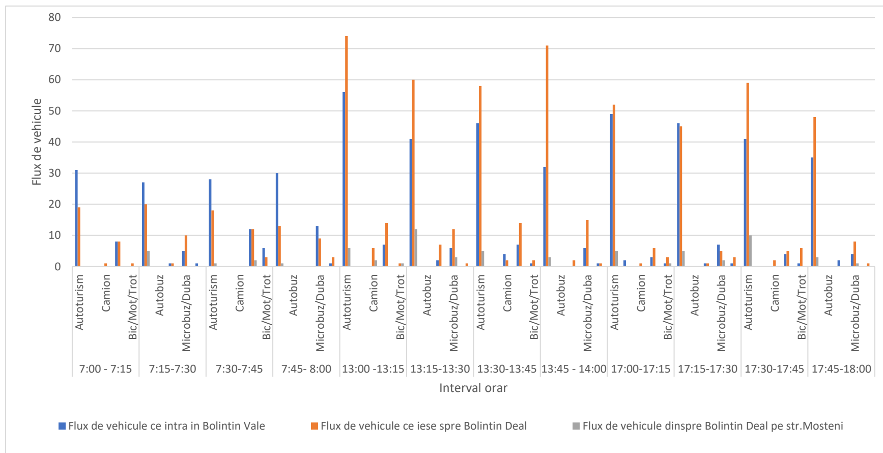
Fig. 3.2.20.a. Flux de vehicule intrare / ieșire în Bolintin Vale / spre Bolintin Deal (Camera 1.3.2)
