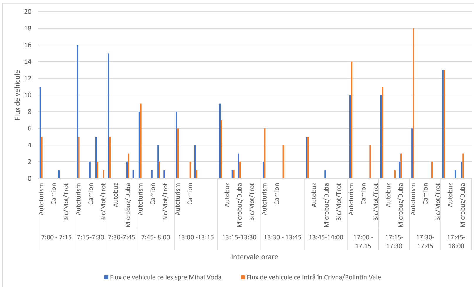
Fig. 3.2.21. Fluxul de vehicule ce intră în Crivina, respectiv care ies în direcția Mihai Vodă (Camera 3.3.1)
