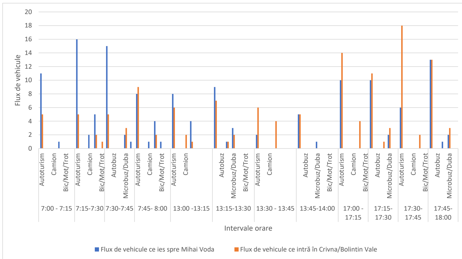
Fig. 3.2.14. Fluxul de vehicule ce intră în Crivina, respectiv care ies în direcția Mihai Vodă (Camera 3.3.1)
