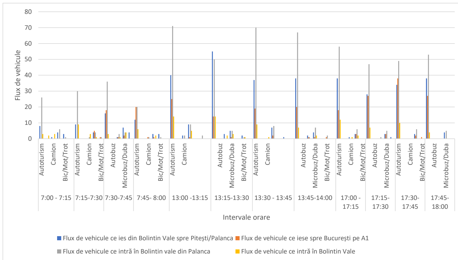
Fig. 3.2.18. Fluxul de vehicule care intră și ies din Bolintin Vale – punctul de monitorizare km 30 (Camera 1.3.3)
