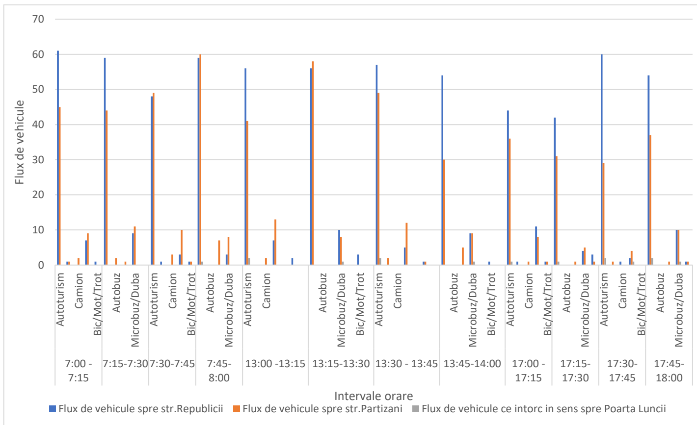
Fig. 3.2.17.a. Fluxul de vehicule care intră / ies în /din sensul giratoriu la intersecția străzilor Poarta Luncii, Partizani și Republicii – acces din strada Poarta Luncii (Camera 1.161)
