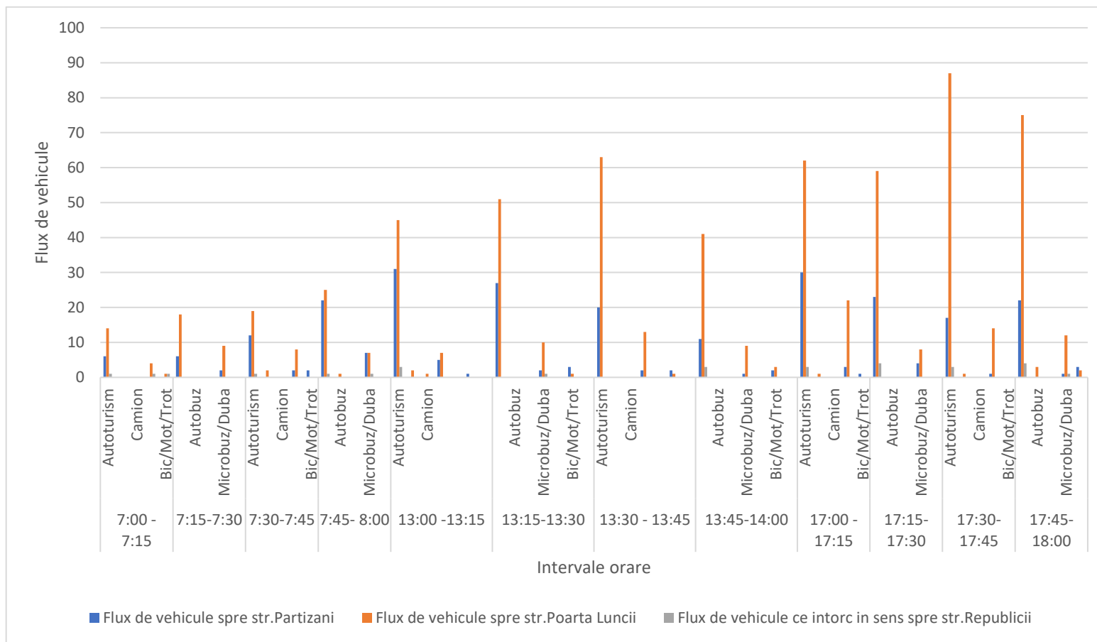
Fig. 3.2.17.b. Fluxul de vehicule care intră / ies în /din sensul giratoriu la intersecția străzilor Poarta Luncii, Partizani și Republicii – acces din strada Republicii (Camera 1.161)
