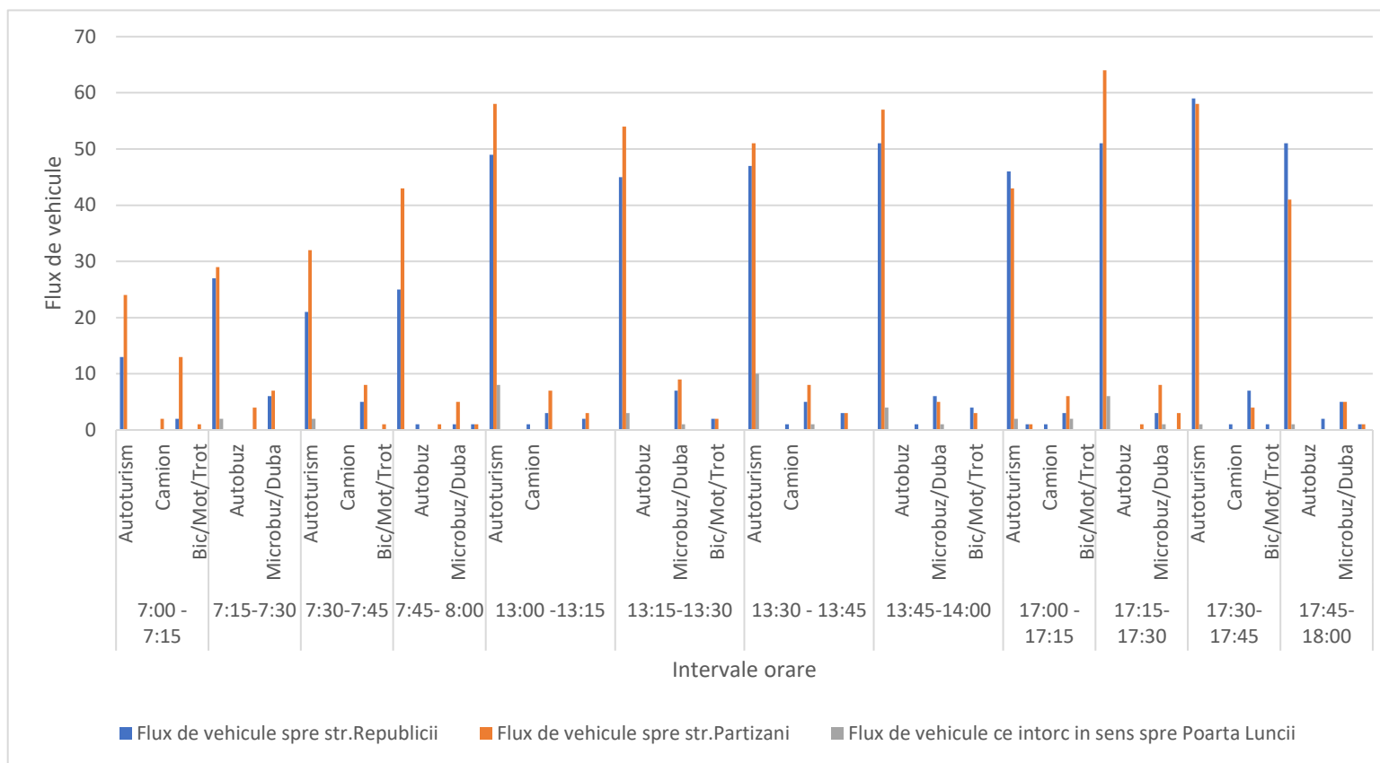
Fig. 3.2.24.a. Fluxul de vehicule care intră / ies în /din sensul giratoriu la intersecția străzilor Poarta Luncii, Partizani și Republicii – acces din strada Poarta Luncii (Camera 1.161)
