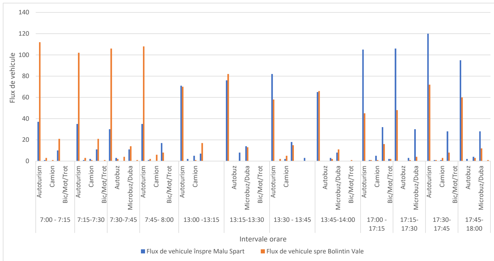
Fig. 3.2.16. Fluxul de vehicule ce se deplasează spre Malu Spart, respectiv ce intră în Bolintin Vale – punct de monitorizare Poarta Luncii (Camera 1.3.1)
