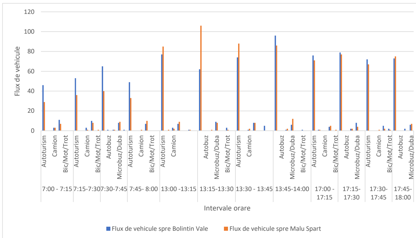
Fig. 3.2.26. Fluxul de vehicule care intră în Bolintin Vale și ies spre Malu Spart – DJ 610 (Camera 2.1.10)
