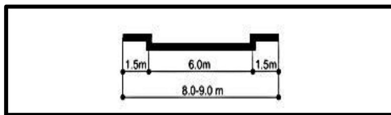
Fig.2.2.7 Profil pentru străzile de categoria IV – de folosință locală (sursa: [12])
