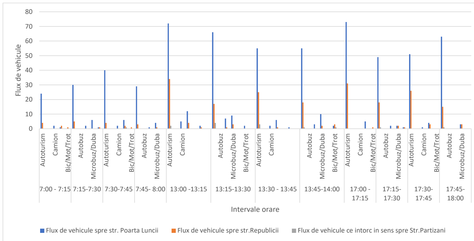
Fig. 3.2.24.c. Fluxul de vehicule care intră / ies în /din sensul giratoriu la intersecția străzilor Poarta Luncii, Partizani și Republicii – acces din strada Poarta Luncii (Camera 1.161)
