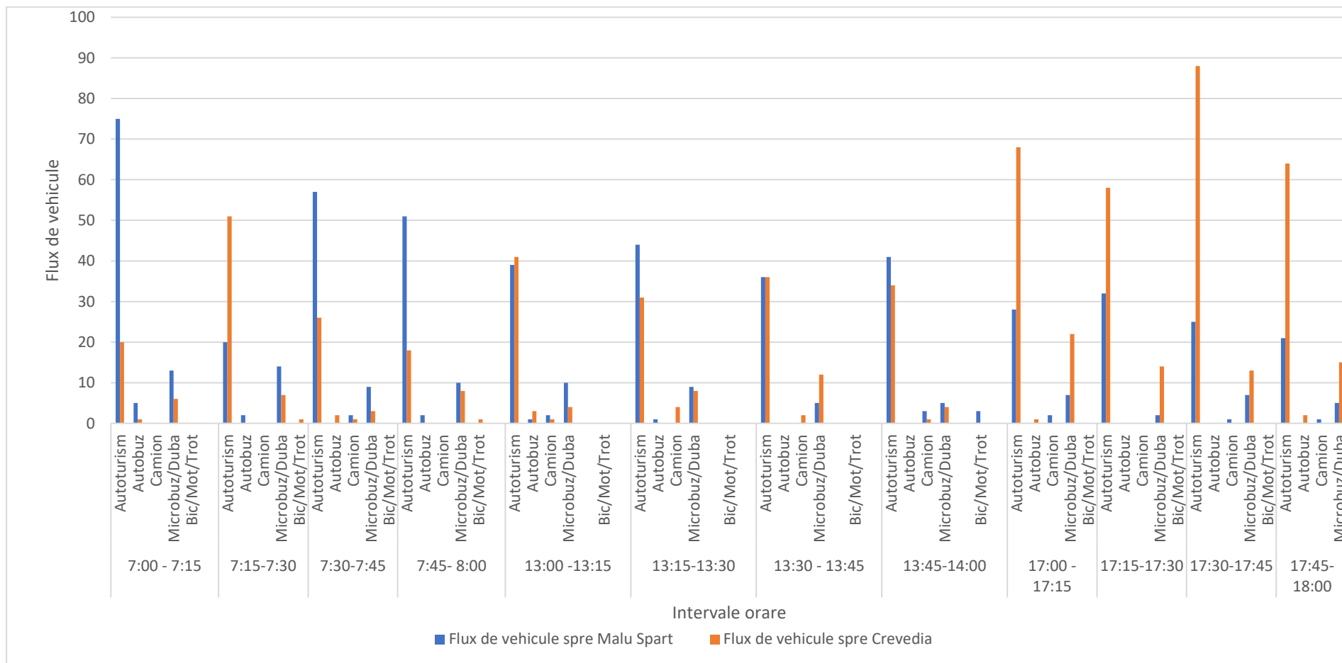
Fig. 3.2.15. Fluxul de vehicule ce se deplasează spre Malu Spart, respectiv Crevedia – punct de monitorizare Ocolul Silvic (Camera 2.3.2)
