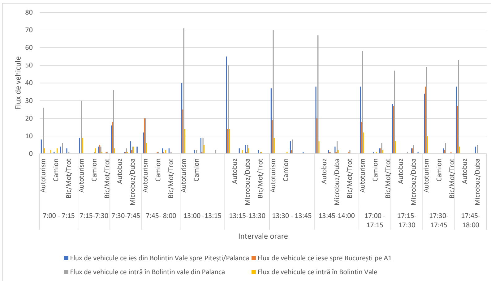
Fig. 3.2.25. Fluxul de vehicule care intră și iese din Bolintin Vale – punctul de monitorizare km 30 (Camera 1.3.3)
