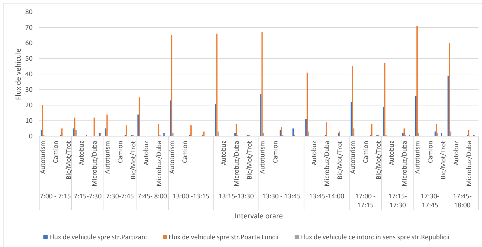
Fig. 3.2.24.b. Fluxul de vehicule care intră / ies în /din sensul giratoriu la intersecția străzilor Poarta Luncii, Partizani și Republicii – acces din strada Republicii (Camera 1.161)
